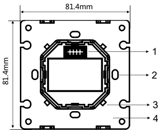
图 2. 尺寸图 - 正面
