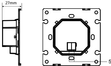
图 3. 尺寸图 - 侧面
