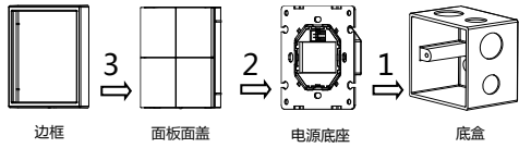
图 5. 安装图
