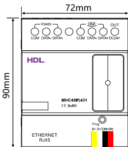
图 2. 尺寸图 - 正面
