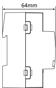
图 3. 尺寸图 - 侧面
