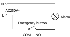
图 6. 接线图
