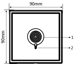
图 3. 尺寸图 - 正面 带金属边框
