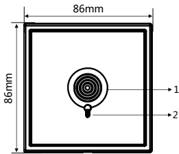
图 2. 尺寸图 - 正面 带塑料边框
