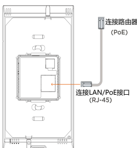
图 5. 网络连接
