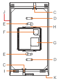
图 4. 部件 - 背面图 (带不锈钢垫片)
